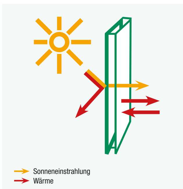
ISOLAR SOLARLUX® in Sommerfunktion.
